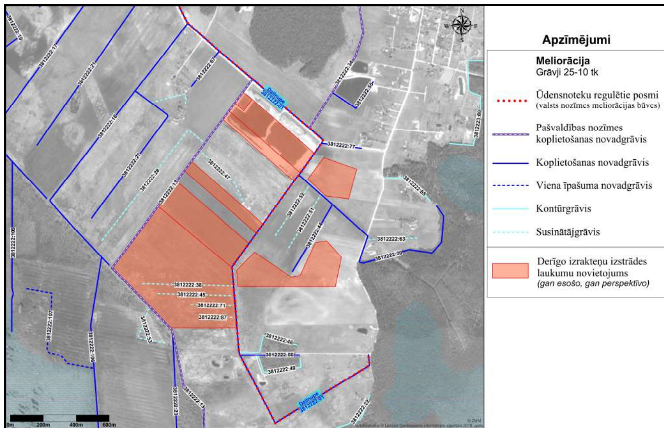
Attēls Nr.2 Meliorācijas sistēmu shēma Atradnei pieguļošajā teritorijā (Avots: Valsts meliorācijas kadastrs)
