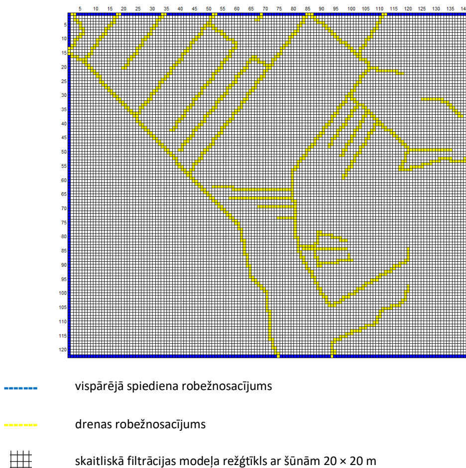
Attēls Nr.24 Hidroģeoloģiskā modeļa režģītīks un filtrācijas robežnosacījumi
