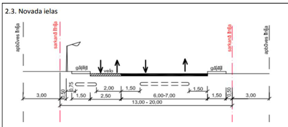
Attēls Nr.3 Novada ielas (tai skaitā V-21) šķēršprofils (Avots: Mārupes novada teritorijas plānojuma 2014. – 2026.gadam Teritorijas izmantošanas un apbūves noteikumi, 1.pielikums)
